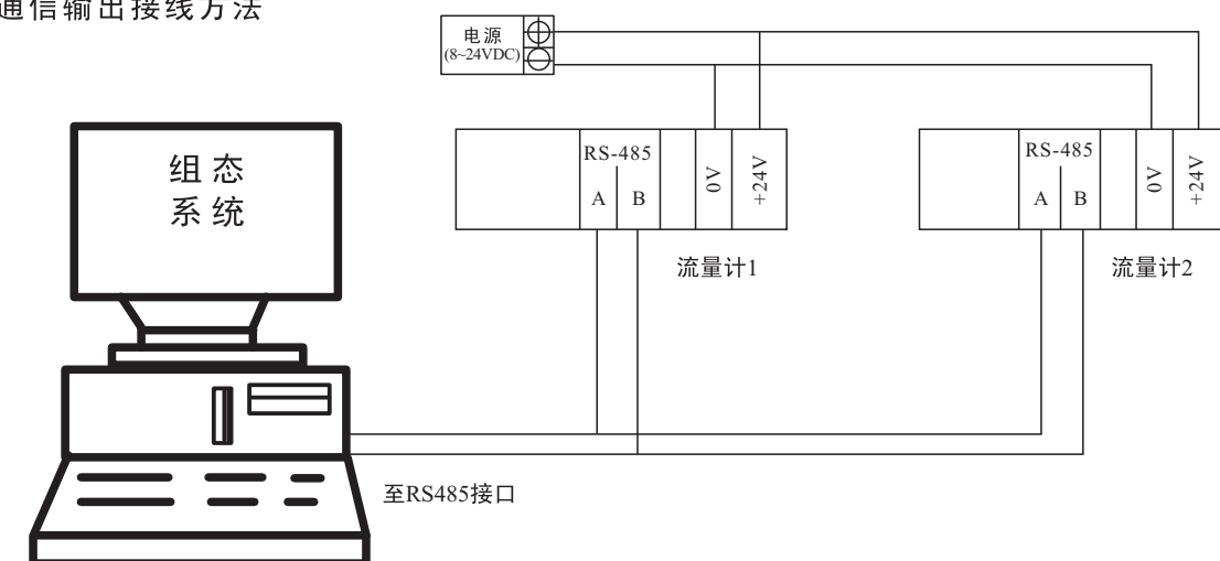
f. 通信输出接线方法
