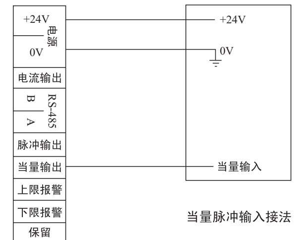
d. 当量输出接线方法
